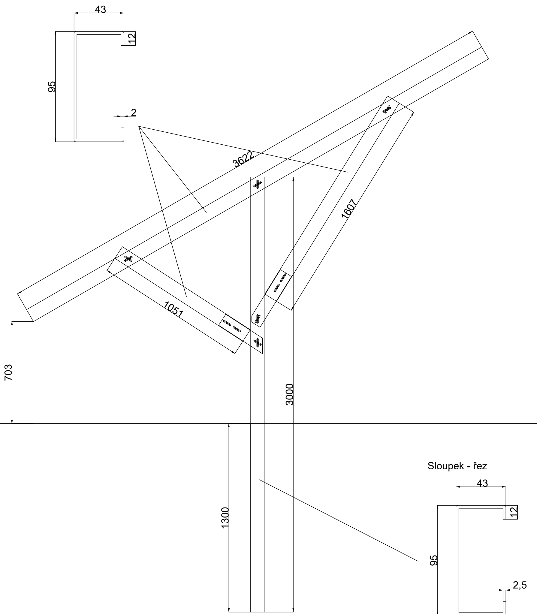
Hlavní profil a vzpěry - řez
